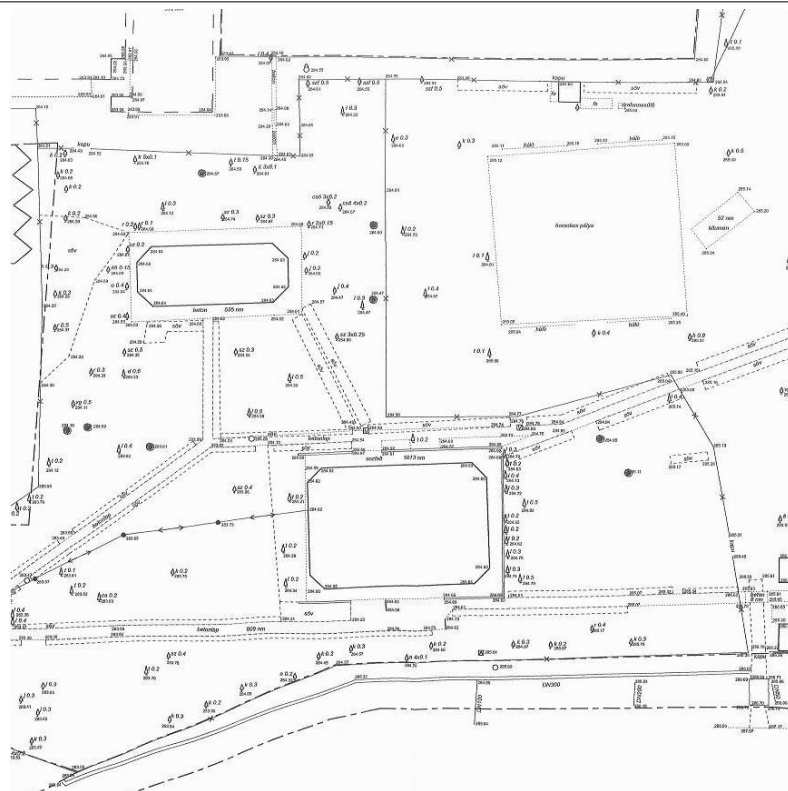
2. ábra – Helyszínrajz felmérés
