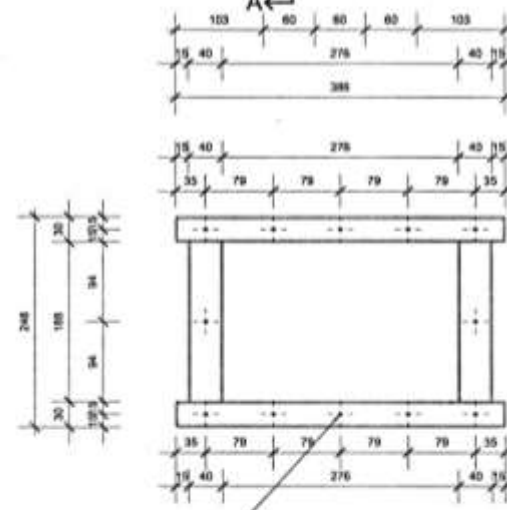
DOMBORMŰ VB. KERETEZÉS FELRÖGZÍTÉSE, ELŐLNÉZET M = 1 : 50
