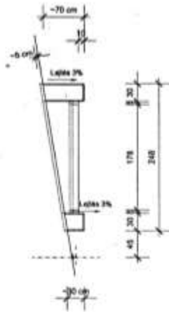
DOMBORMŰ FELRÖGZÍTÉSE A-A FÜGGŐLEGES METSZET M = 1 : 50
